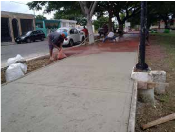
Construcción de banquetas y guarniciones en la colonia Lindavista, Mérida, Yuc. 2010 INCCOPY
